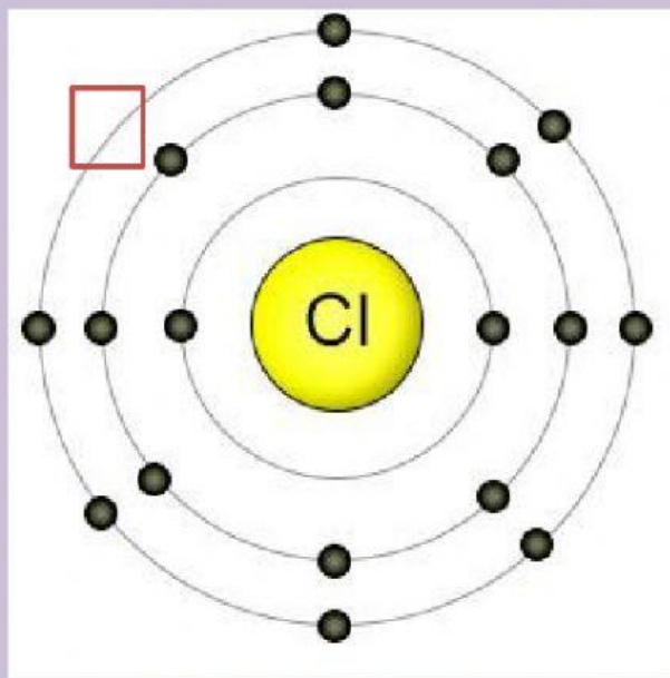
Fig 2 : CHLORINE
