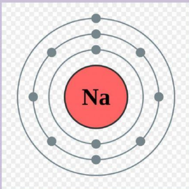
Fig 1 : SODIUM
