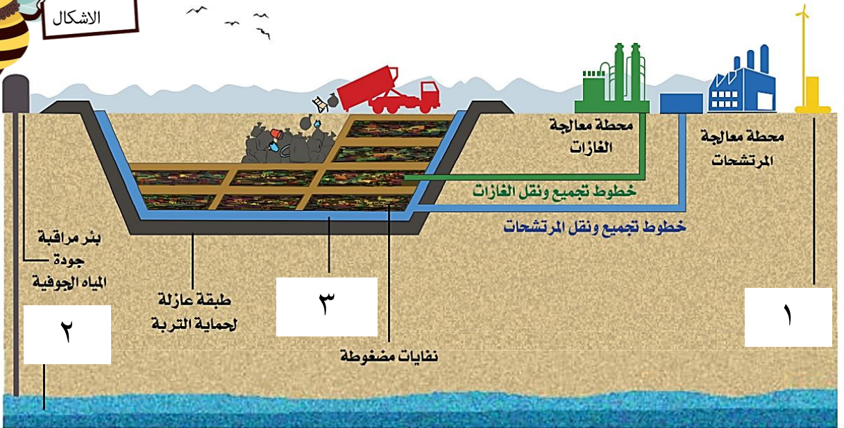
الشكل (٨) رسم توضيحي لمردم هندسي
