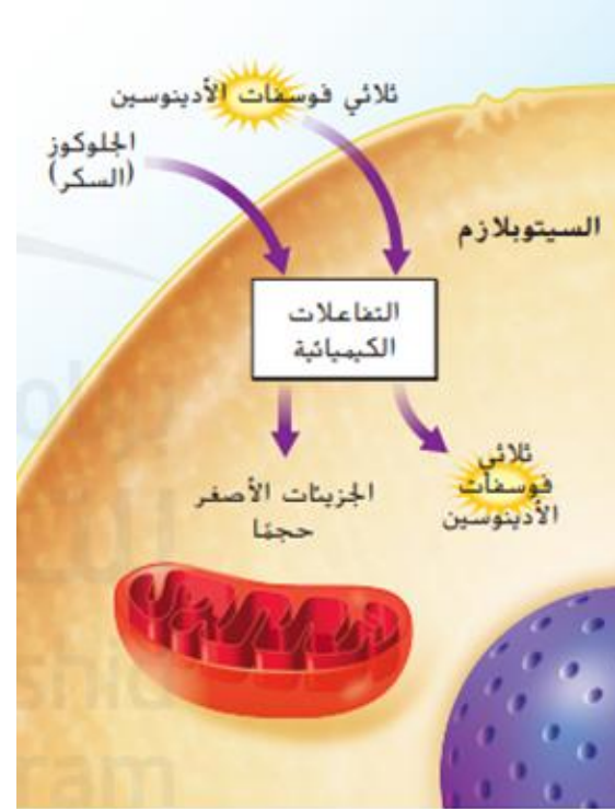
الشكل 15 يمثل التحلل السكري أولى خطوات التنفس الخلوي.
