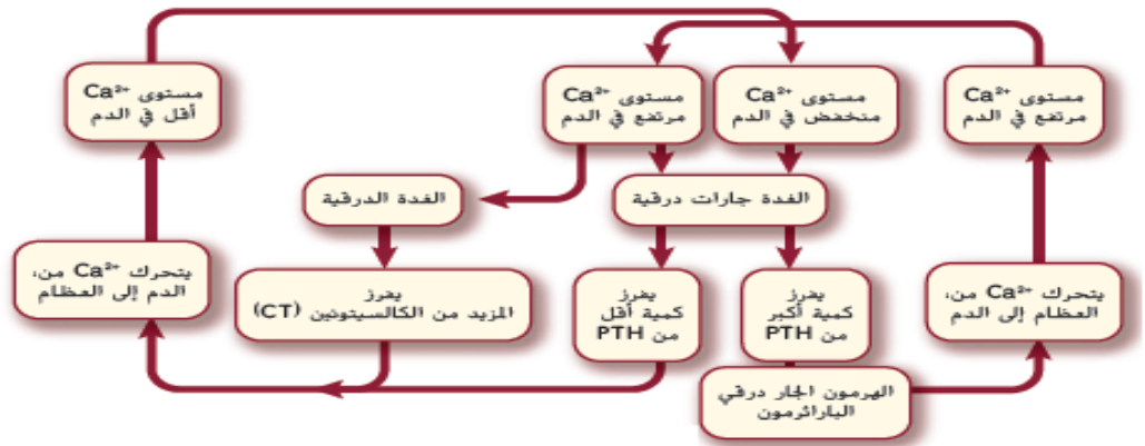
الشكل 17 يُنظم الهرمون الجاردرقي (PTH) وهرمون الكالسيتونين (CT) مستوى الكالسيوم في الدم. أشرح كيف يوضح هرمون الباراثورمون (PTH) وهرمون الكالسيتونين (CT) الآلية الراجعة السلبية.
