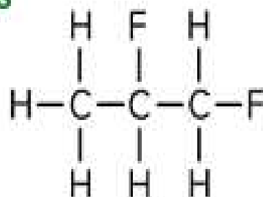
1,2-Difluoropropane
