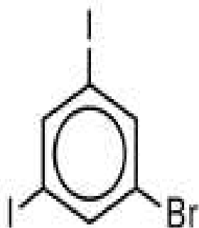
1-Bromo-3,5-diiodobenzene
