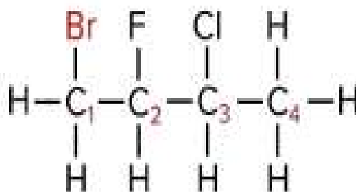
1-Bromo-3-chloro-2-fluorobutane
