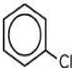
Chlorobenzene
