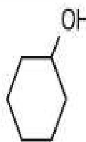
Cyclohexanol
