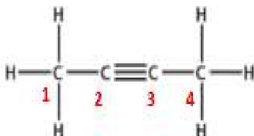
2-Butyne
