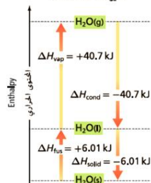
Phase Changes for Water تغيرات حالة الماء
